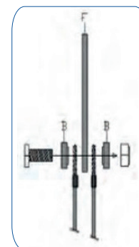
zestaw mocujący KFL do złączy gwintowanych
